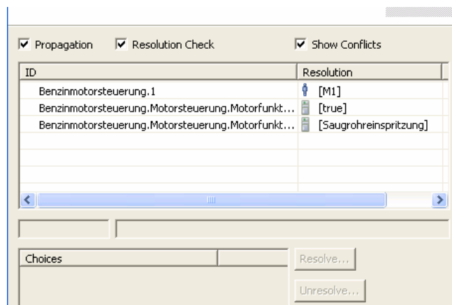
Abbildung 23: Beispiel: Instantiierung
